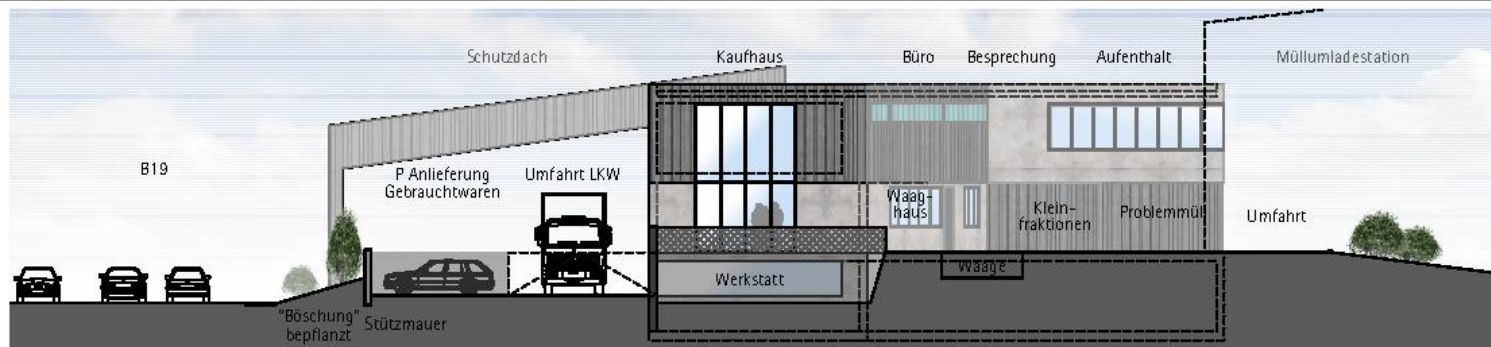
Ansicht Süd
