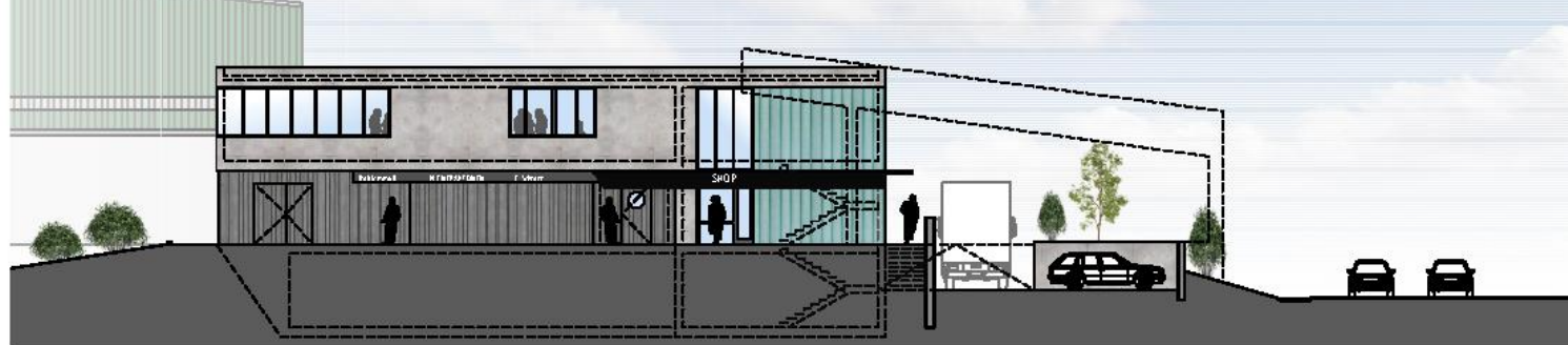
Ansicht Nord
